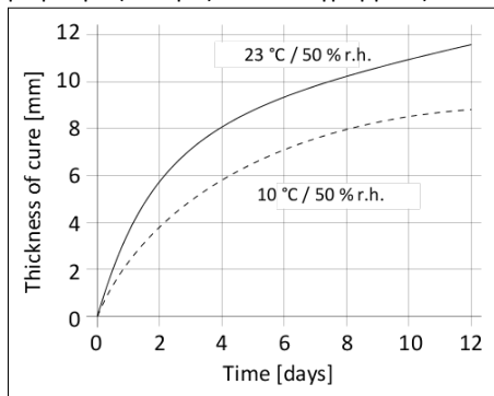
Διάγραμμα 1: Ταχύτητα ωρίμανσης του Sikaflex®-290 DC PRO
